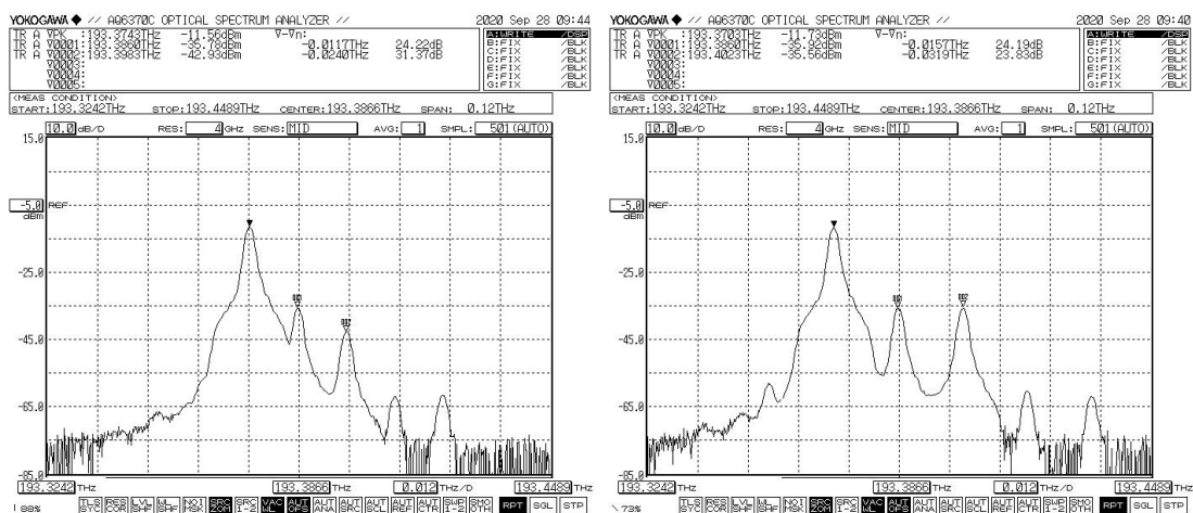
图 2 12GHz 和 16GHz 测试结果
