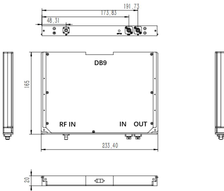
图 3 单边带模块尺寸图 (不含 RF 驱动)
